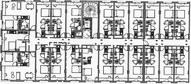
PLAN NIVEAU
