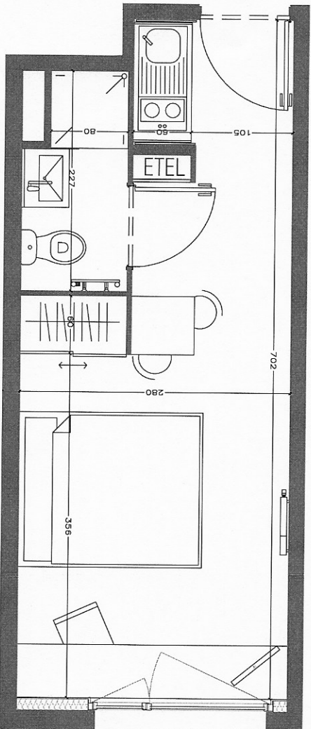
PLAN NIVEAU
